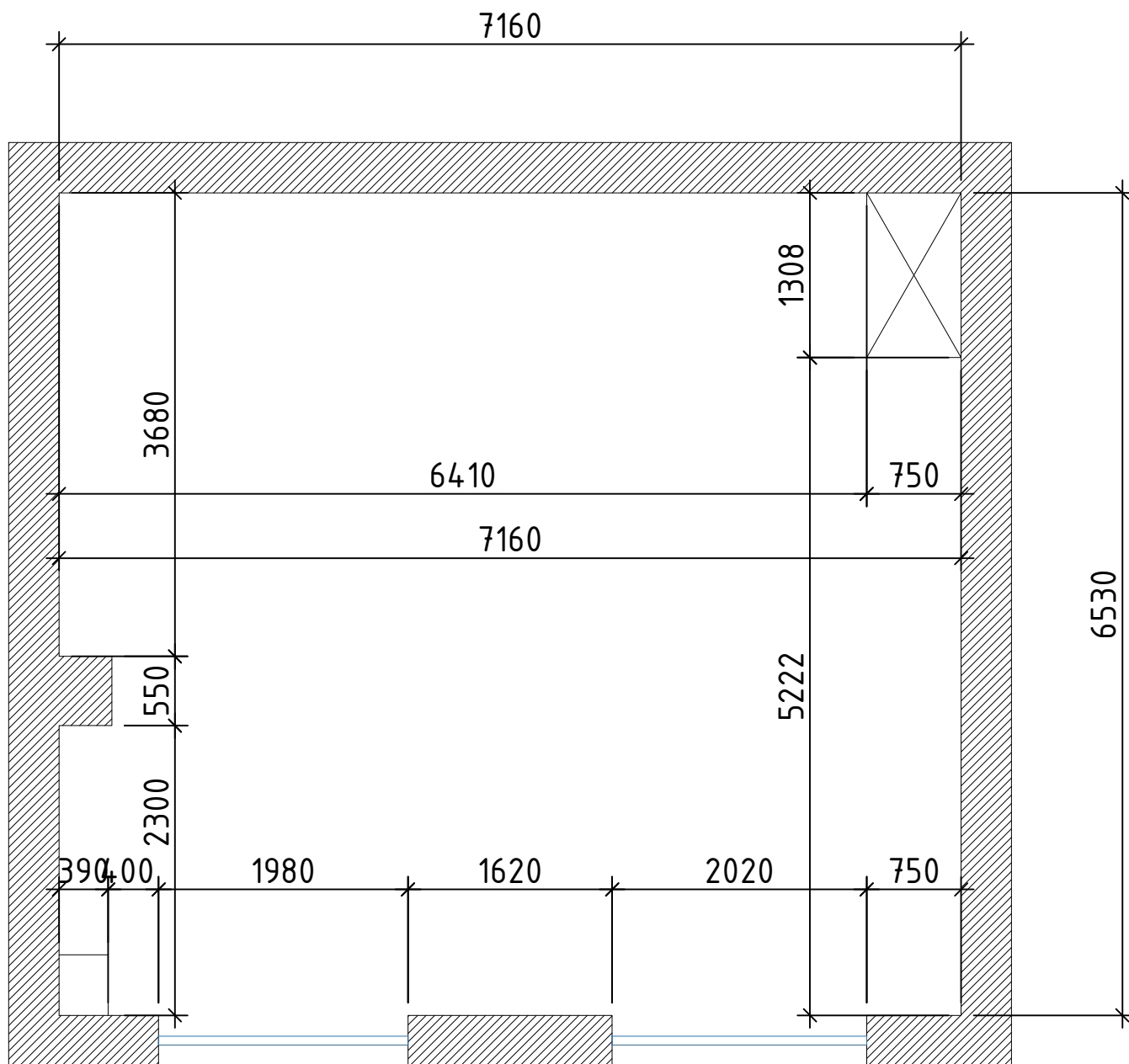
Обмерный план М1:100
